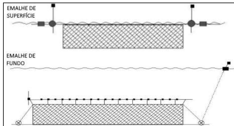
Redes de Emalhe - Fonte: Adaptado de CEPISUL/IBAMA
