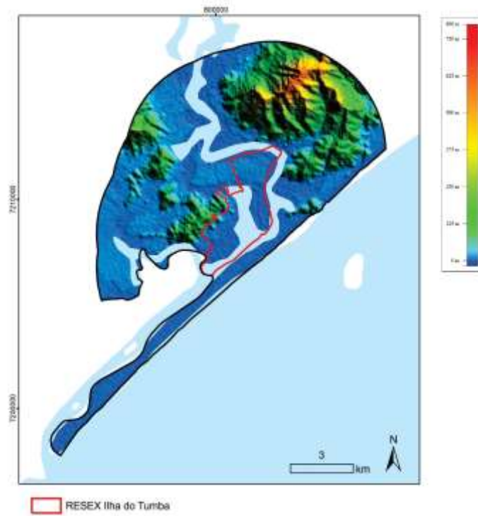
Figura 4- Modelo Digital de Terreno (MDTs) da RESEX ILHA DO TUMBA e sua área de abrangência com base nos dados SRTM (2004).
