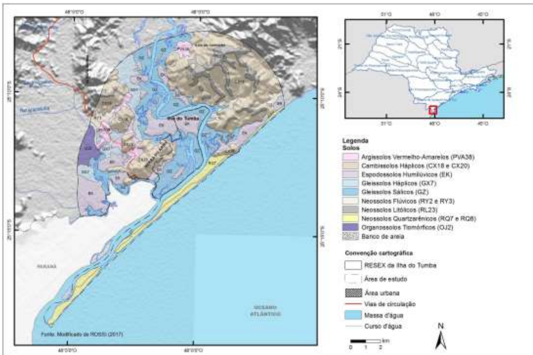
Mapa pedológico da Reserva Extrativista da Ilha do Tumba
