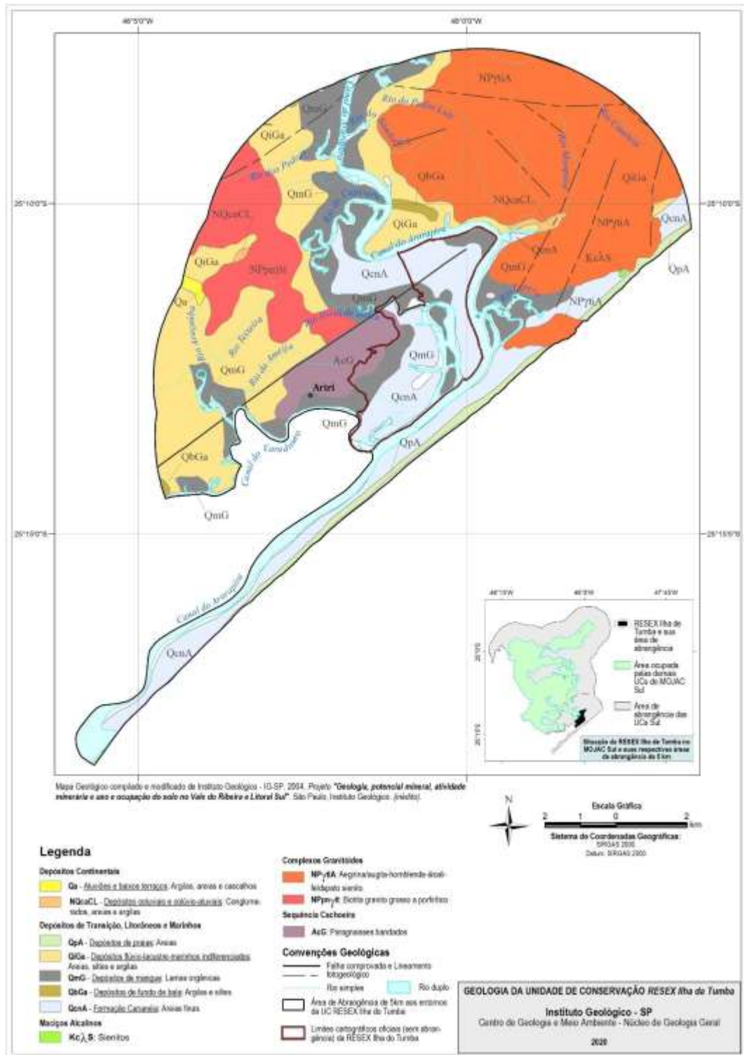
Figura 2: Geologia da Unidade de conservação – RESEX Ilha da Tumba.
